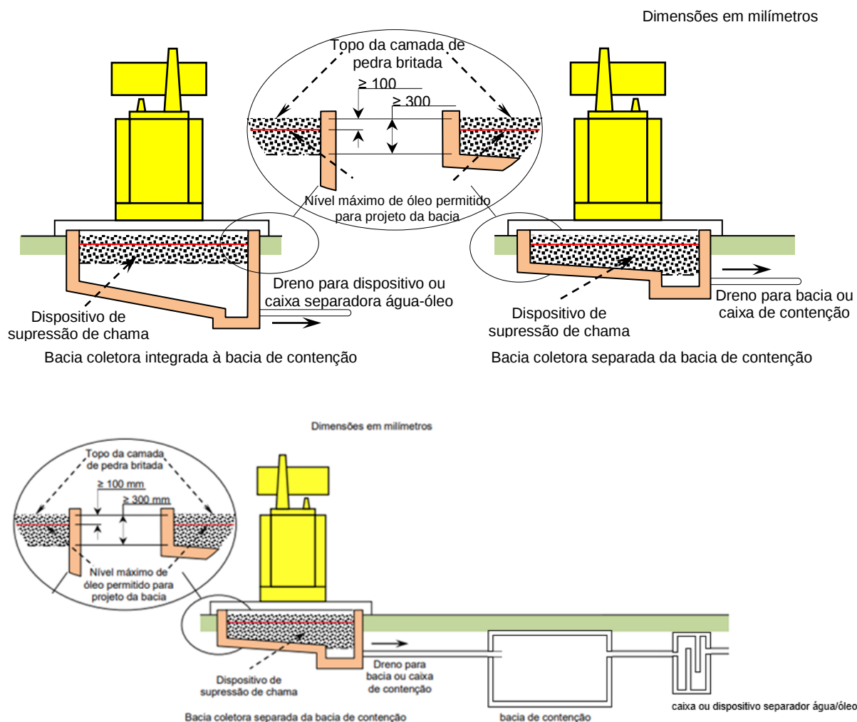
Figura A.6: Exemplo de bacia coletora de contenção e bacia de contenção
