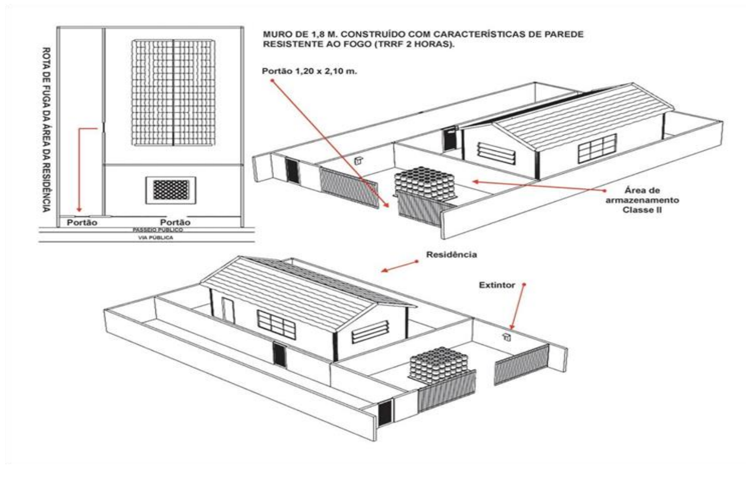
Figura 01: Revendedor classe II com entrada independente
