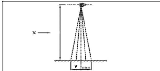
Figura 1: modelo sprinkler – horizontal ( side wall ) para cortina d'água. (valores x, y, respectivamente altura de instalação e comprimento linear de cobertura do jato, conforme catálogo do fabricante).
