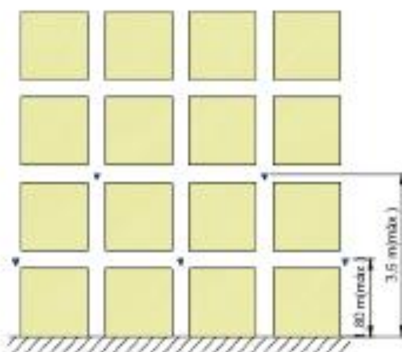
Elevação lateral
