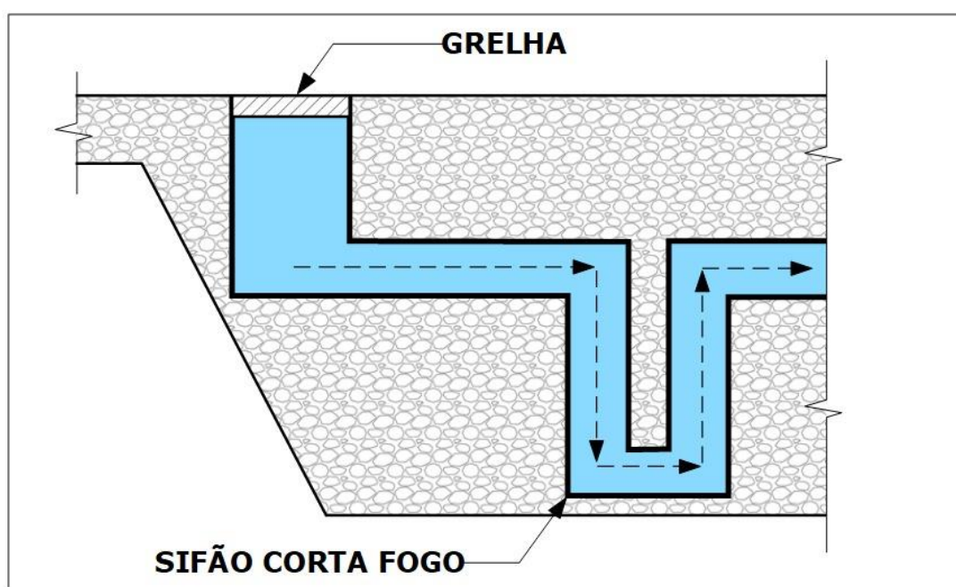
Figura 4.1C: Detalhes do projeto de drenagem de canaletas.
