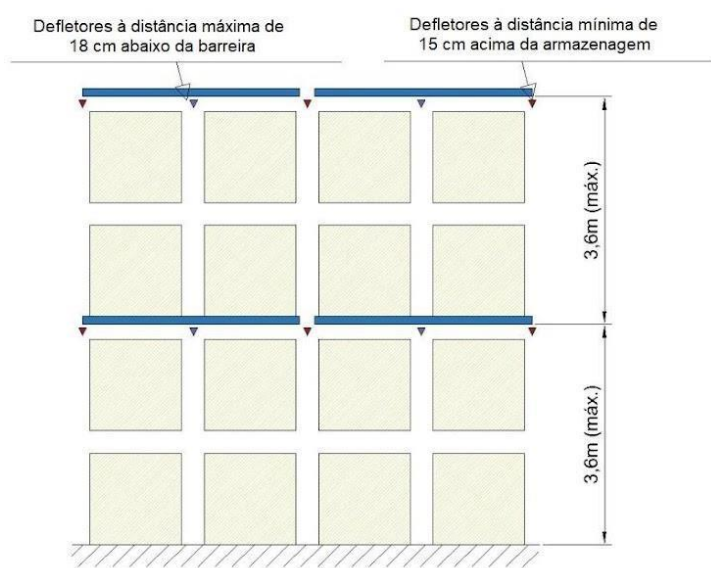
Elevação
