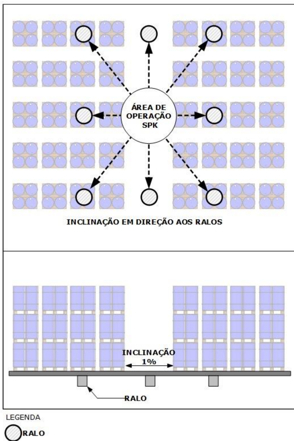
Figura 4.1D: Arranjo típico de drenos de piso.
