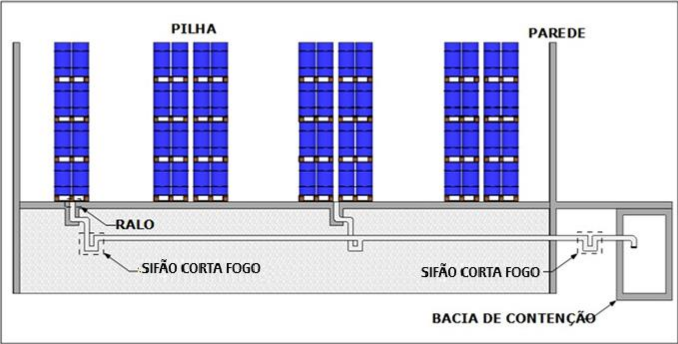
Figura 4.1A: Esquema geral para controle de derramamentos de líquidos em armazéns.
