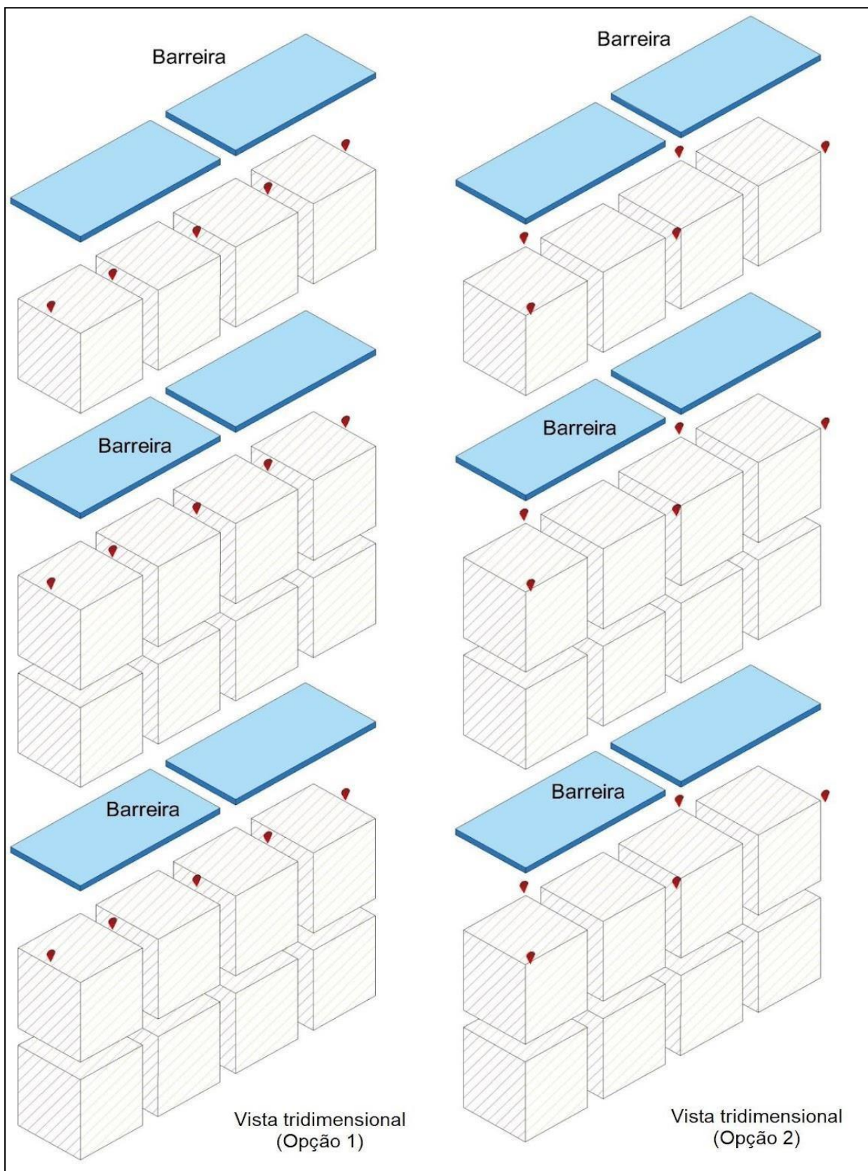
Figura 4.12 Leiaute de chuveiros automáticos para estrutura-suporte de fileira única – Esquema de projeto "C".
