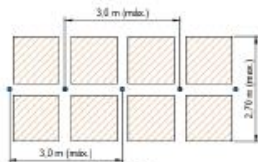
Planta baixa
