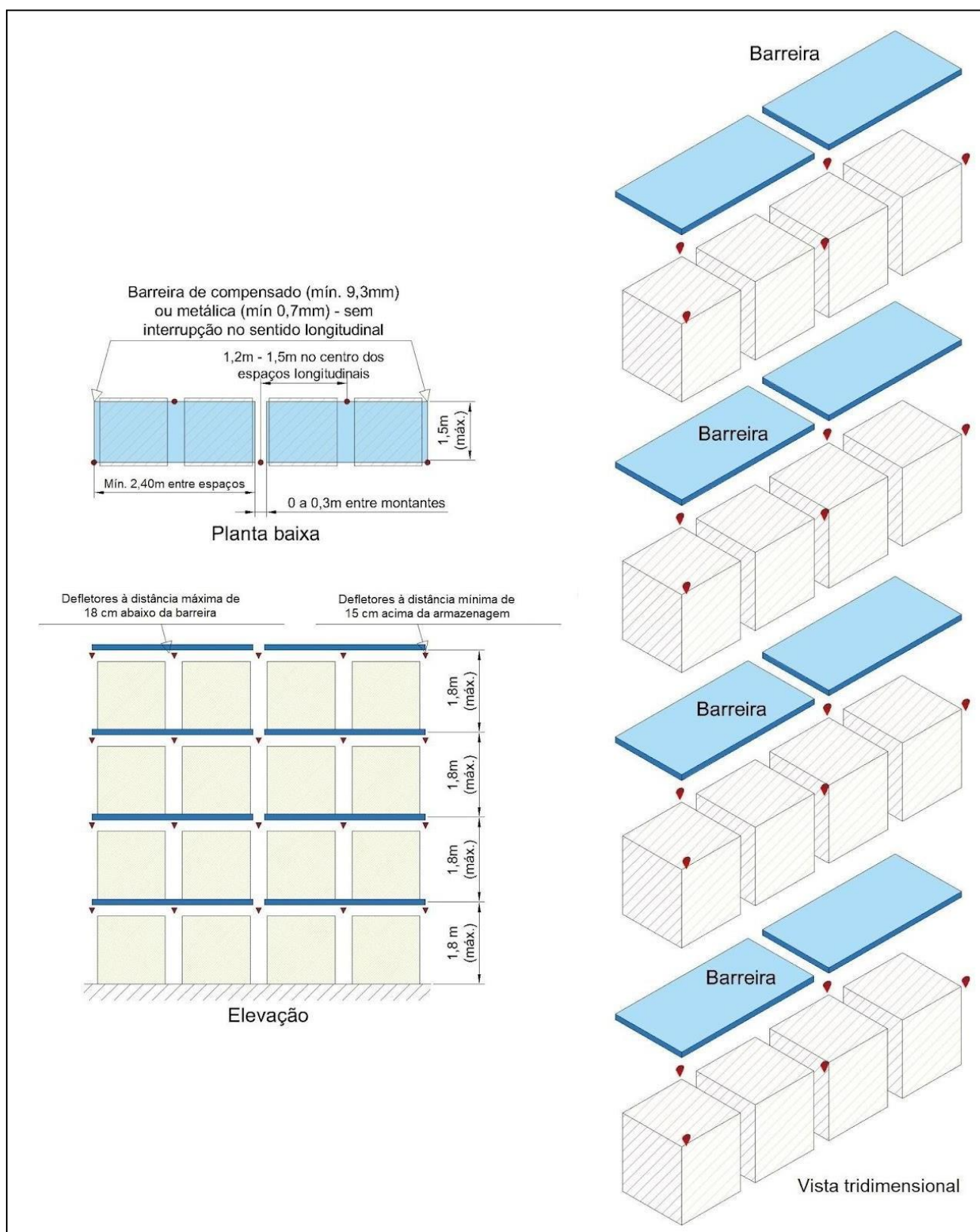
Figura 4.10: Leiaute de chuveiros automáticos para estrutura-suporte de fileira única – Esquema de projeto “B” – Chuveiros voltados para a estrutura.
