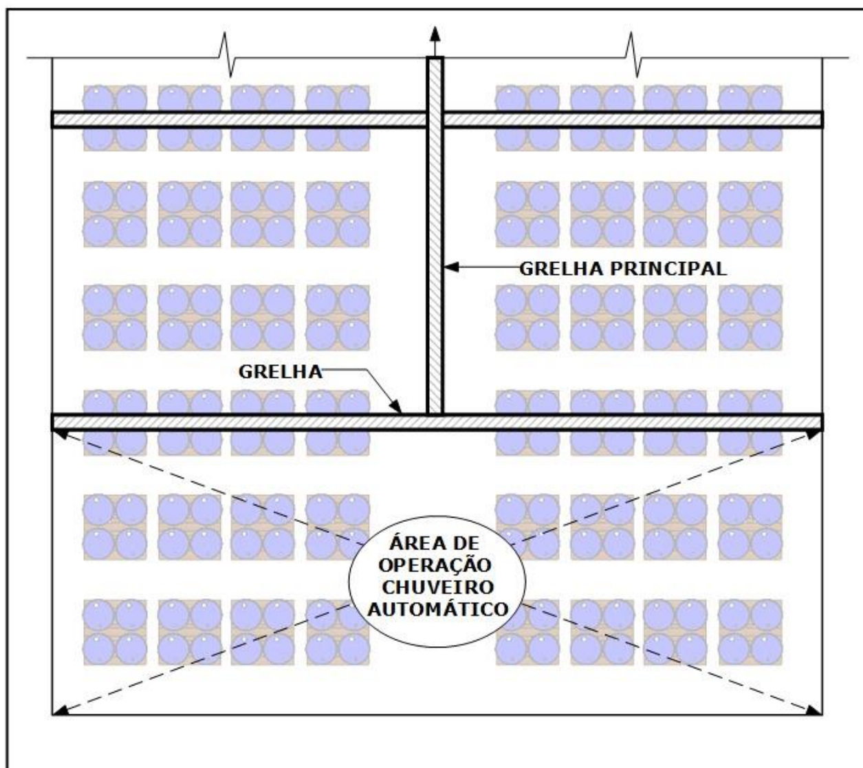
Figura 4.1B: Vista em planta de controle de líquidos em armazéns.
