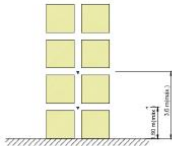
Elevação frontal
