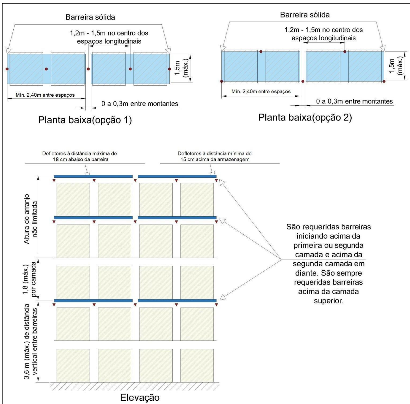
Figura 4.12: Leiaute de chuveiros automáticos para estrutura-suporte de fileira única – Esquema de projeto "C". (continua)
