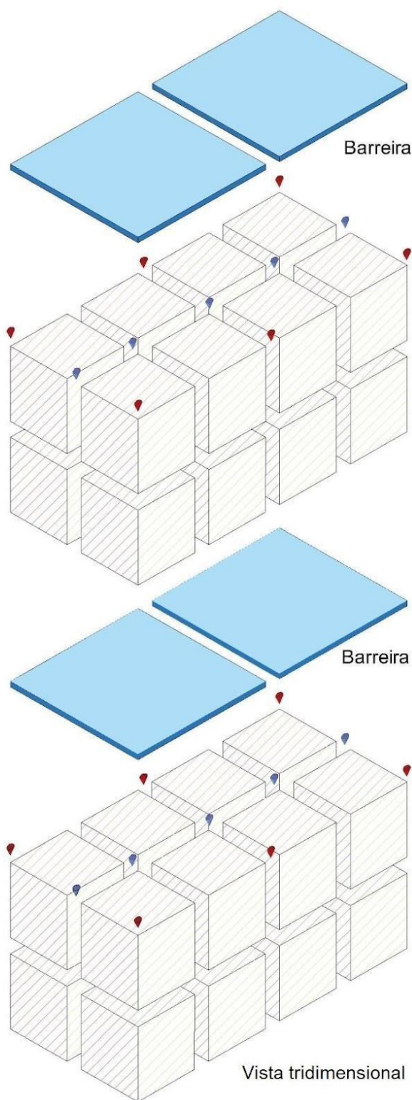
Figura 4.7: Layout de chuveiros automáticos para uma estrutura-suporte de madeira dupla – Esquema de projeto "A"
