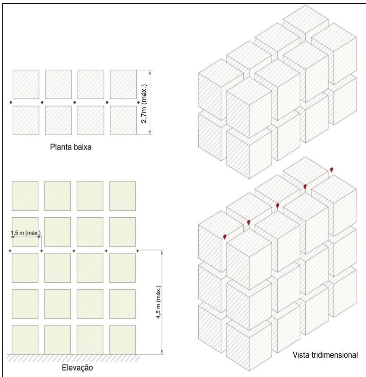
Figura 4.19: Leiaute de chuveiros automáticos para estrutura-suporte de fileira dupla – Leiaute “H” - Opção # 2.
