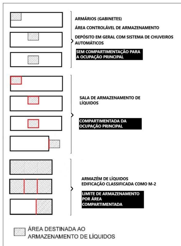
Figura 4.1: Exemplos das modalidades de armazenamento.
