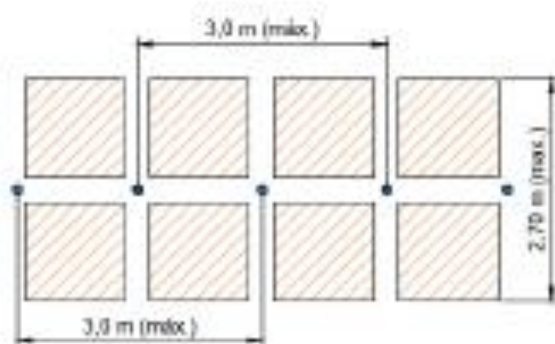
Planta baixa
