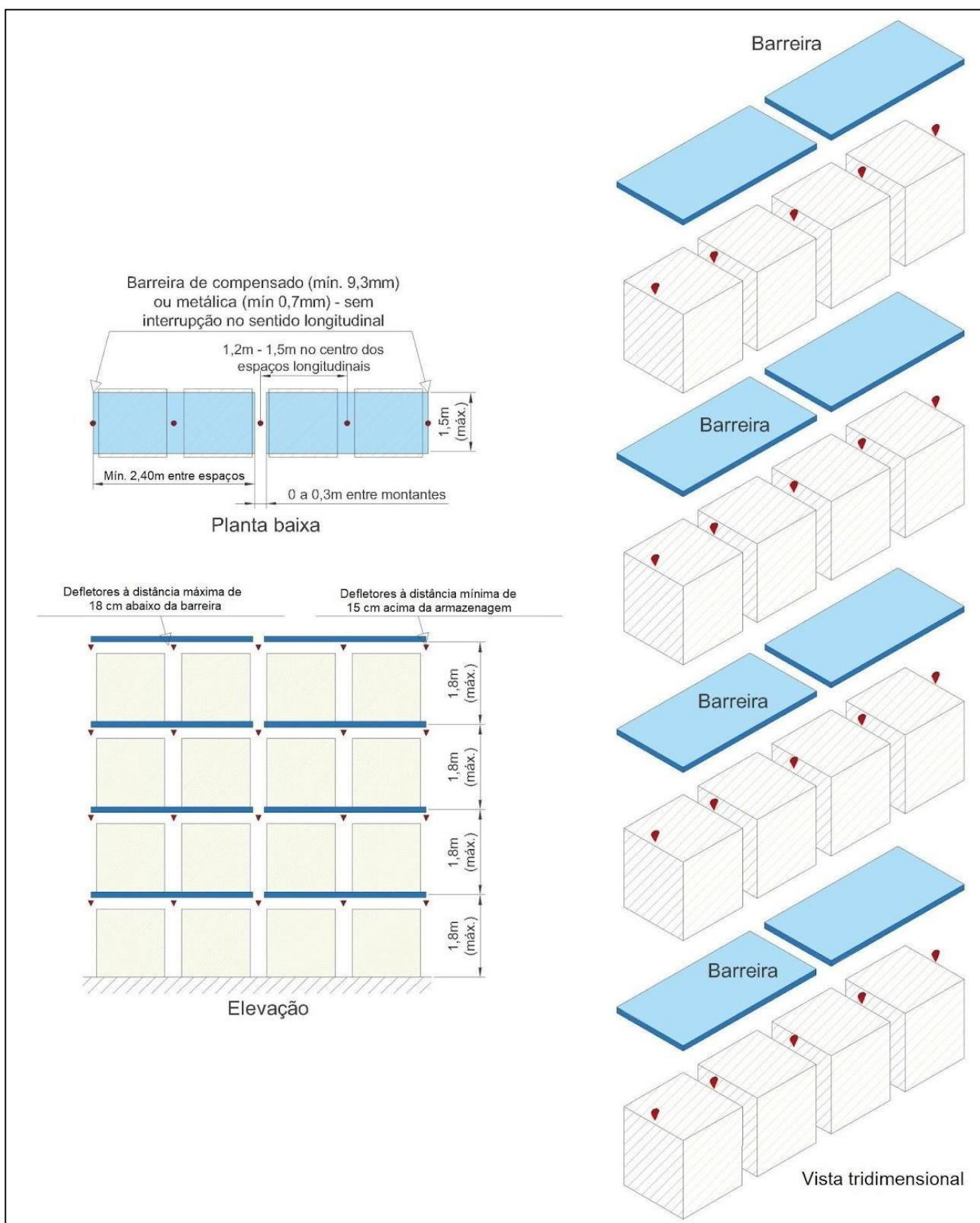
Figura 4.9: Leiaute de chuveiros automáticos para estrutura-suporte de fileira única Esquema de projeto “B” – Chuveiros no centro da estrutura.
