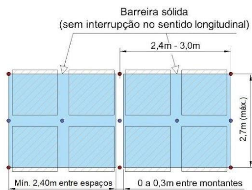
Planta baixa
