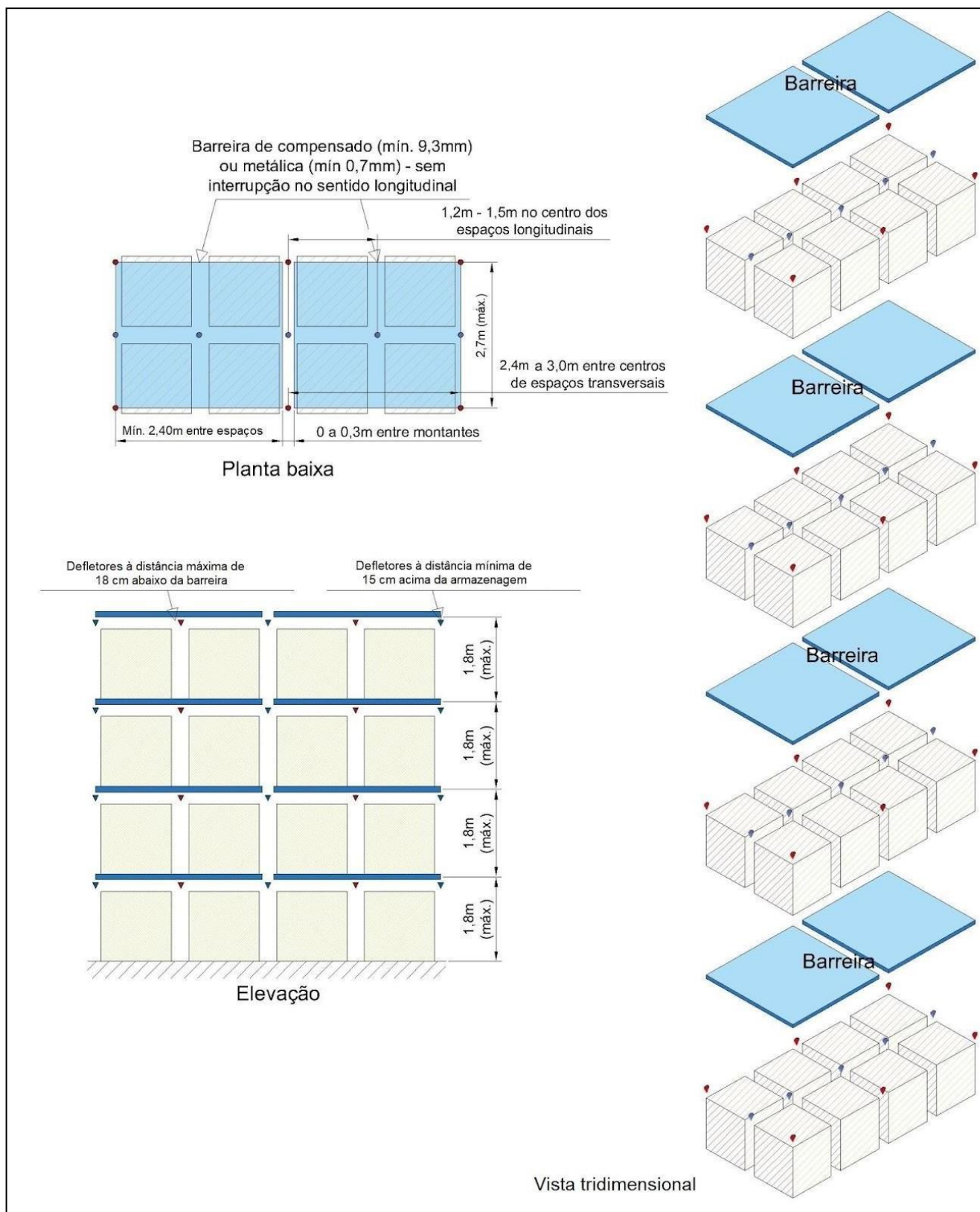
Figura 4.11: Leiaute de chuveiros automáticos para estrutura-suporte de fileira dupla – Esquema de projeto “B”.
