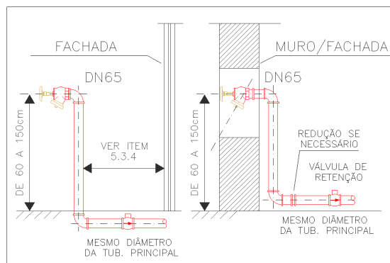
Figura 1: Dispositivo de recalque do tipo coluna para o Corpo de Bombeiros Militar
