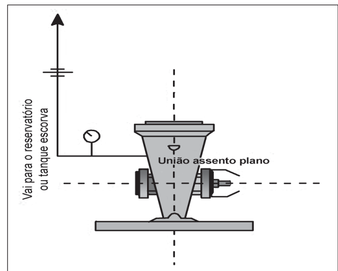
Figura C.7: Arrefecimento da bomba principal elétrica
