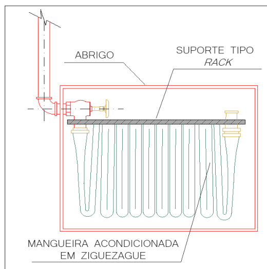
Figura 2: Suporte para mangueira tipo rack
