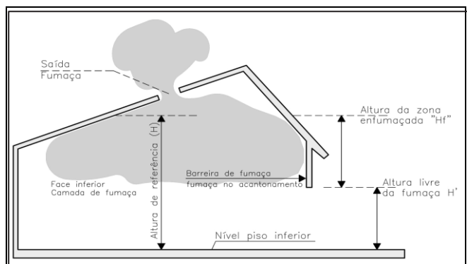
Figura 13: Altura de referência, livre de fumaça e da zona enfumada
