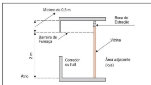
Figura 3: Detalhe de barreira de fumaça – corte
