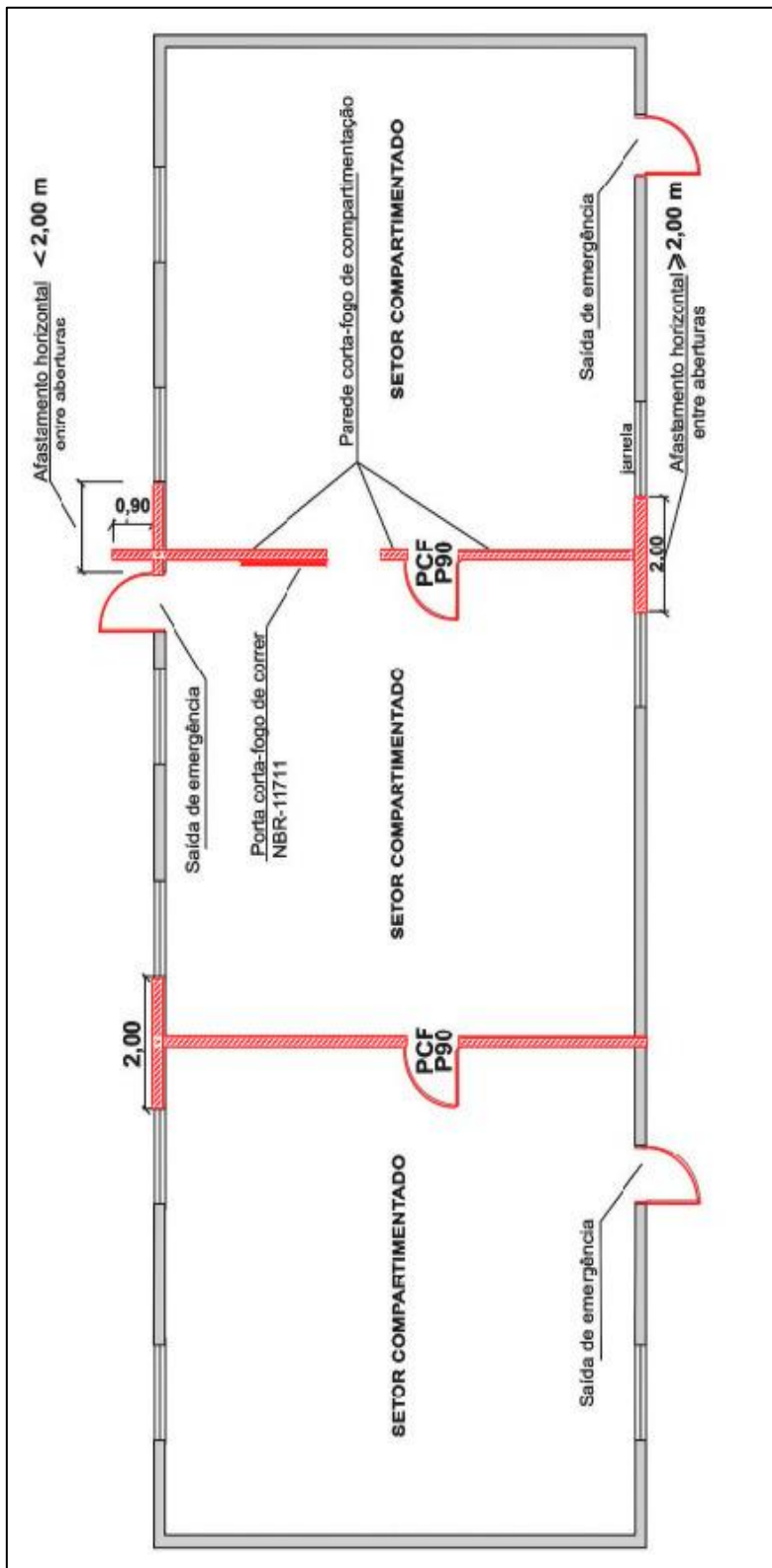
Figura A1: Modelo de compartimentação horizontal
