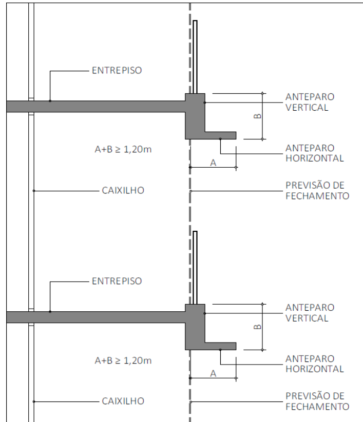
Figura A8: Modelo de fechamento com vidro
