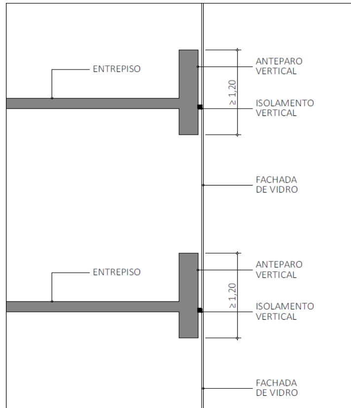
Figura A10: Modelo de compartimentação com fachada envidraçada
