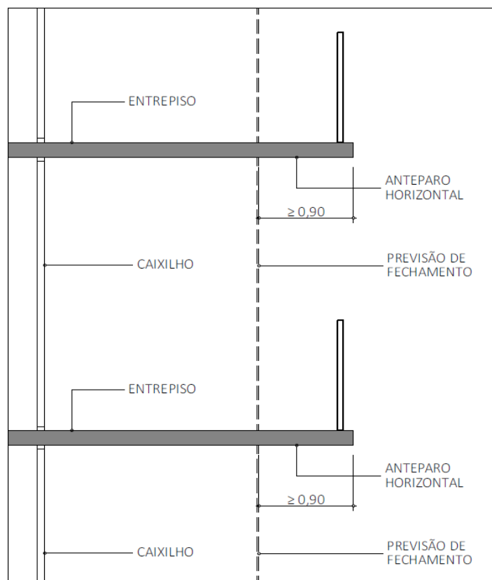
Figura A7: Modelo de fechamento com vidro
