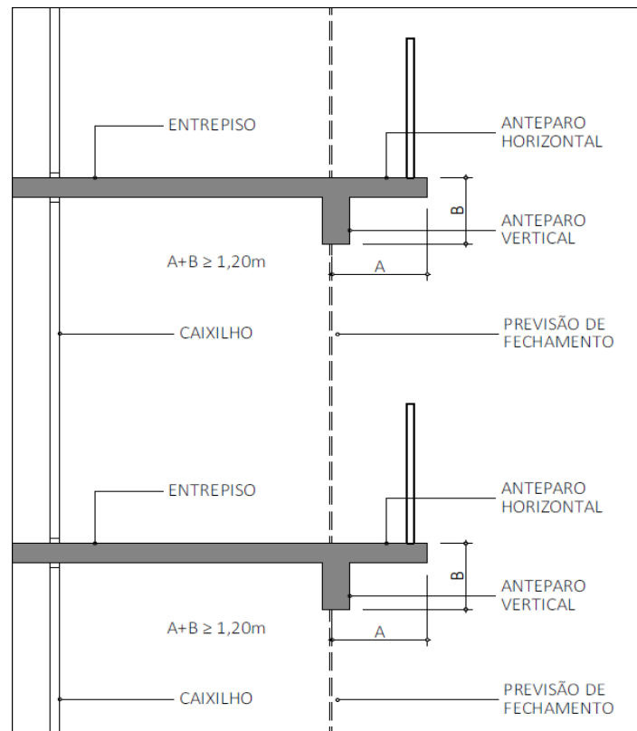
Figura A9: Modelo de fechamento com vidro
