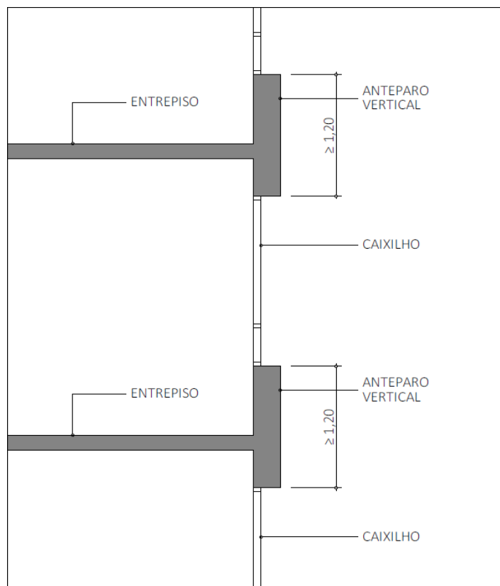
Figura A2: Modelo de compartimentação com anteparo vertical
