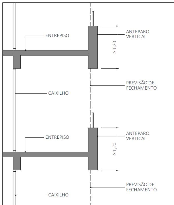
Figura A6: Modelo de fechamento com vidro
