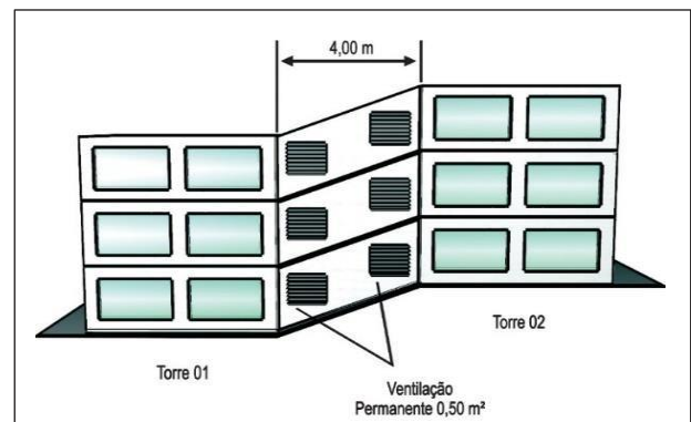
Figura 13: Abertura lateral na escada
