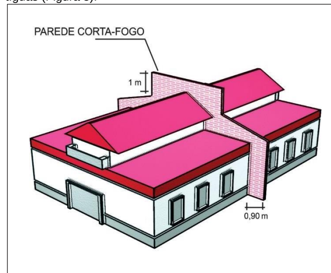
Figura 8: Parede corta-fogo
