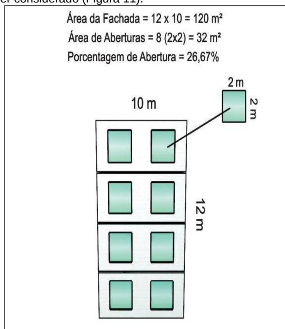
Figura 11: Porcentagem de aberturas na fachada
