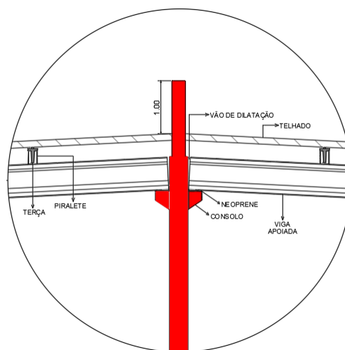
Figura 12: Parede corta-fogo apoiada em consolos (suportes)
