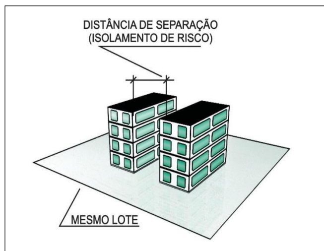
Figura 1: Separação entre edificações no mesmo lote
